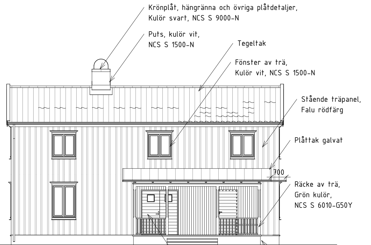
Fasad Framsida, Hustyp 2
