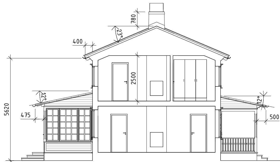
Sektion B-B, Hustyp 2
