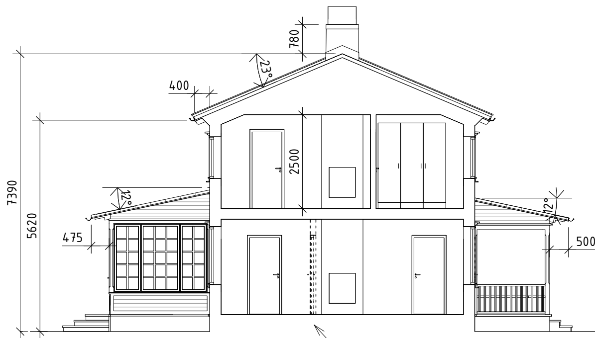
Sektion A-A, Hustyp 1
