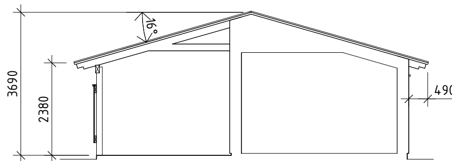
Sektion C-C
